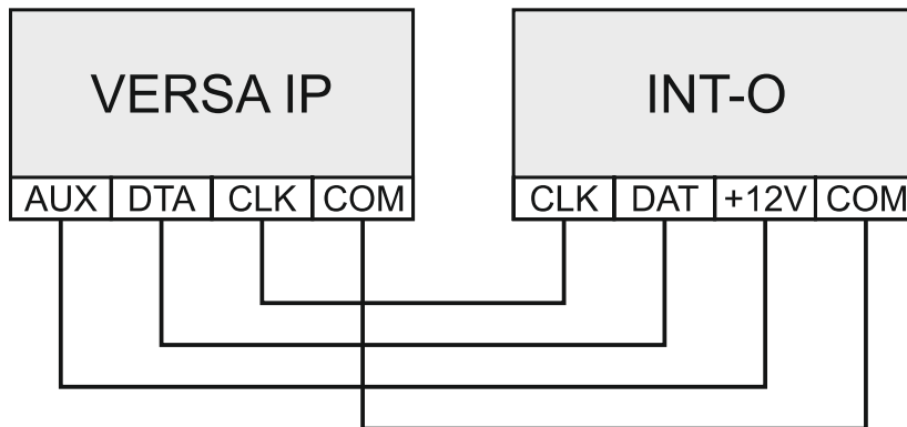
Rys. 13. Sposób podłączenia ekspandera INT-O do centrali.
